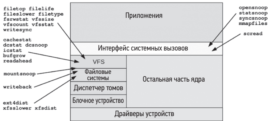
Рис. 8.3. Инструменты BPF для анализа производительности файловых систем
