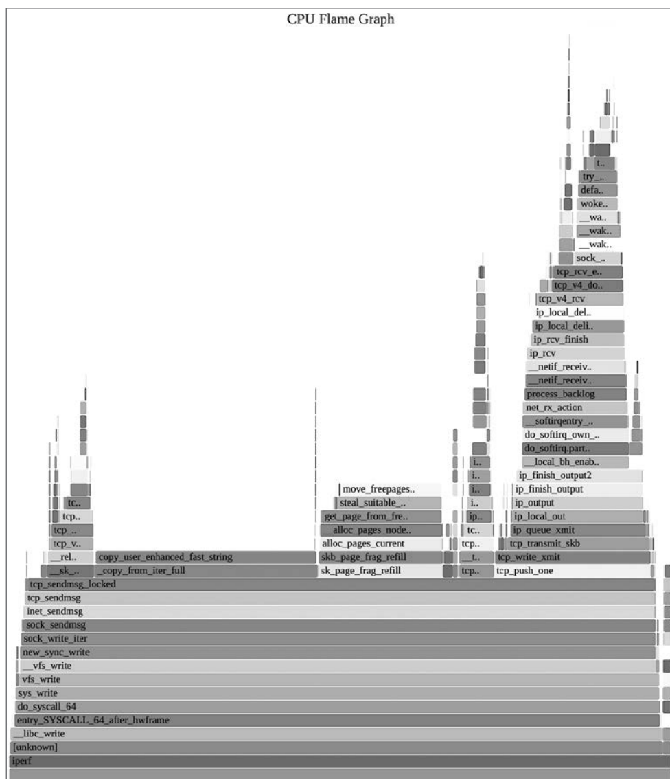
Рис. 6.3. Флейм-график использования CPU
