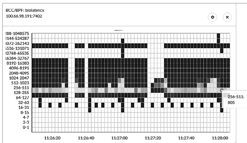
Рис. 17.3. Тепловая карта задержек в Vector, отражающая результаты трассировки с помощью BCC/BPF biol latency(8)
