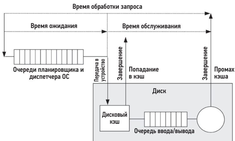
Рис. 9.2. Дисковый ввод/вывод
